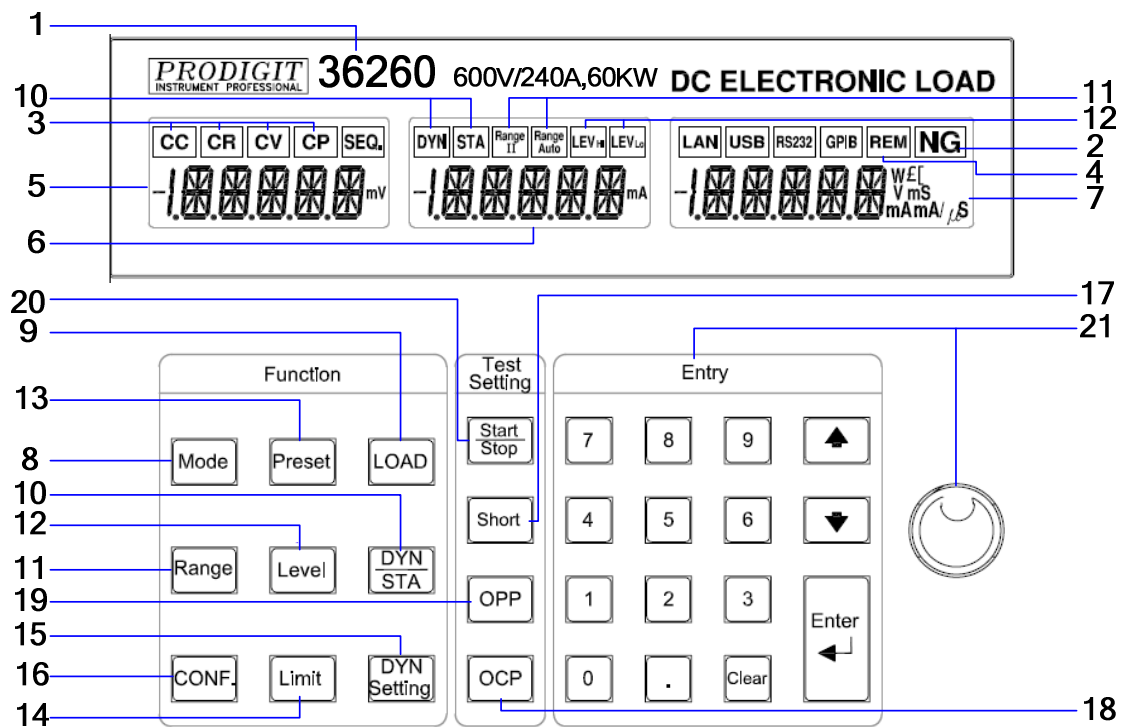
圖 3-4 36000 系列高功率電子負載之面板圖
