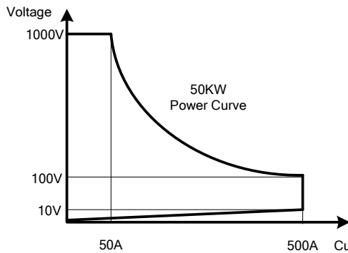
圖 1-1.3 36350高功率電子負載功率曲線圖
