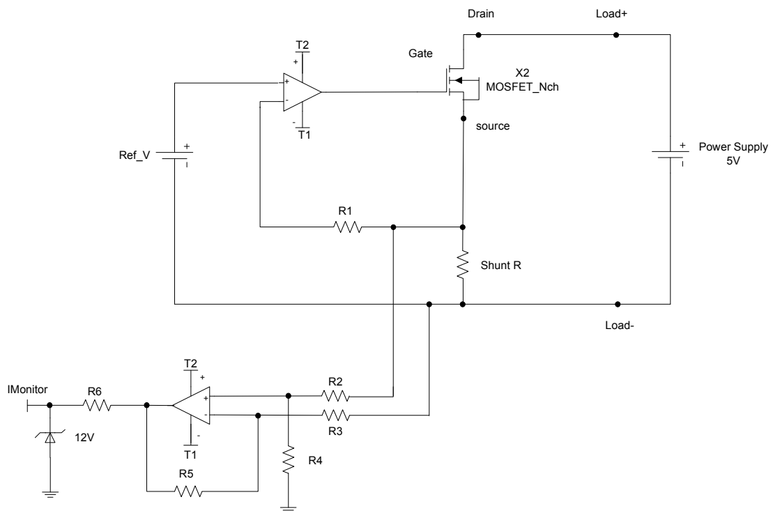
圖 3-6 36000 系列 I-monitor 等效電路圖
