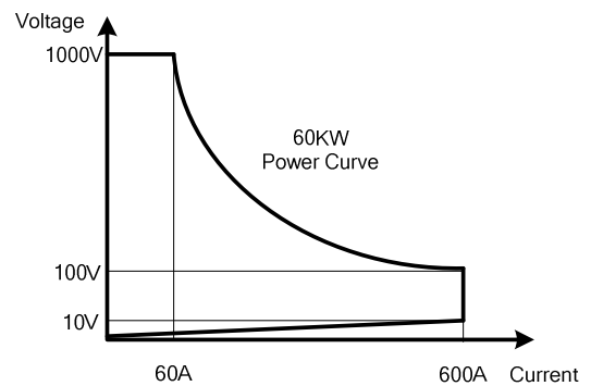
圖 1-1.4 36360高功率電子負載功率曲線圖
