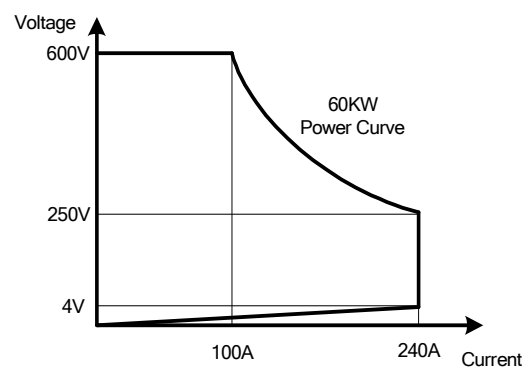
圖 1-1.2 36260高功率電子負載功率曲線圖
