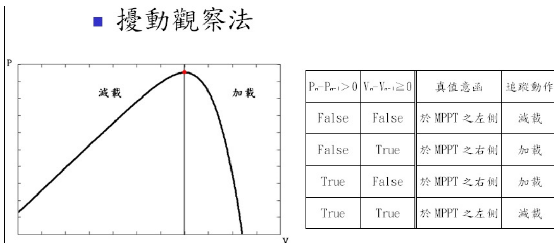
圖 5-12 擾動觀察法動作方式
