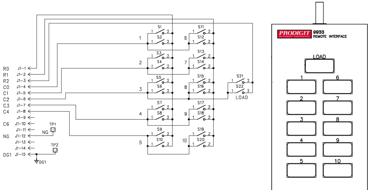
圖 2-9 9933 遙控器連接埠圖
