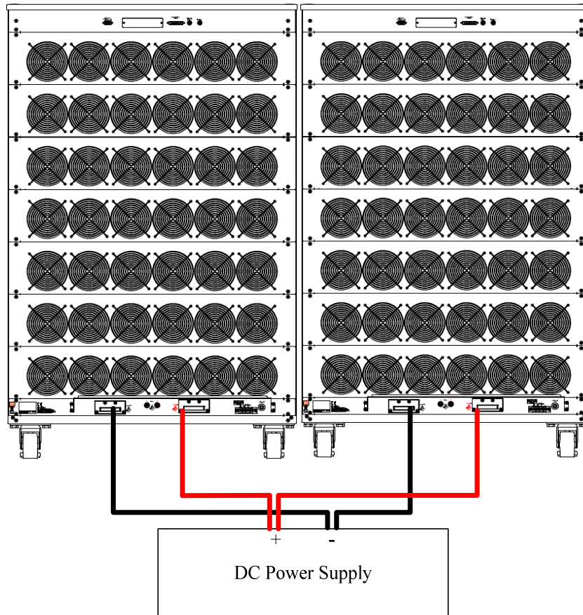
圖 5-10 電子負載多組並聯之連接圖
