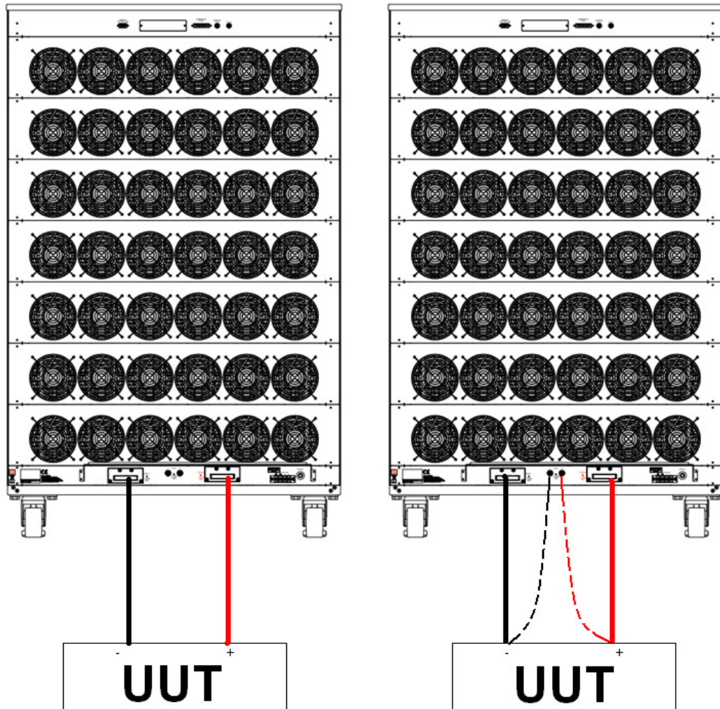
圖 3-5 典型 36000 系列高功率電子負載連接方式
