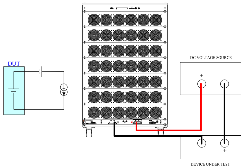
圖 5-9 高功率電子負載最低工作電壓為 0V 時的連接圖
