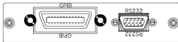
圖 2-2 36000 系列 GPIB & RS232 連接埠圖
