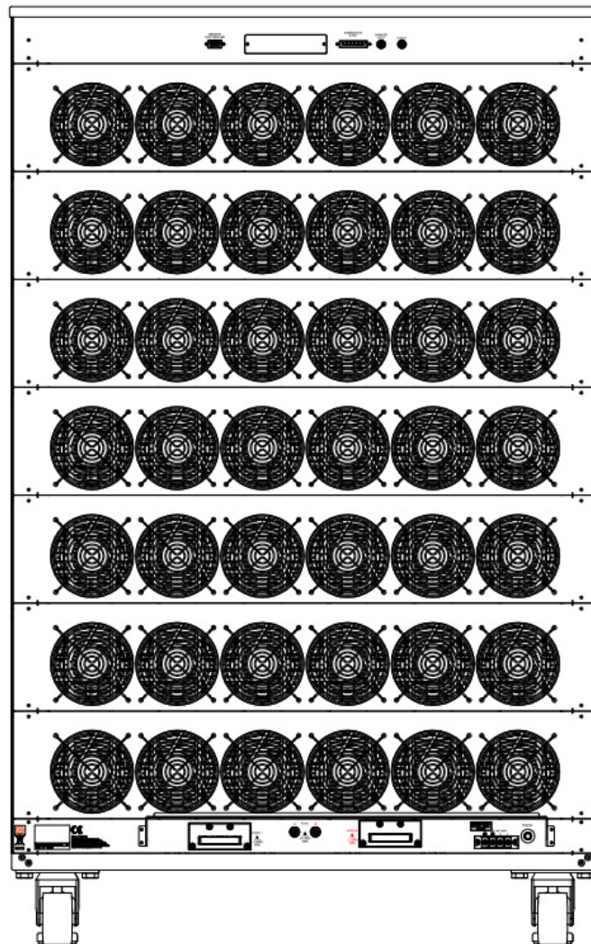
圖 3-2 36000 系列高功率電子負載後面板圖
