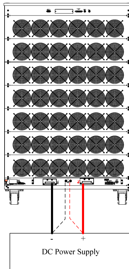
圖 5-2 遠地電壓檢知連接圖
