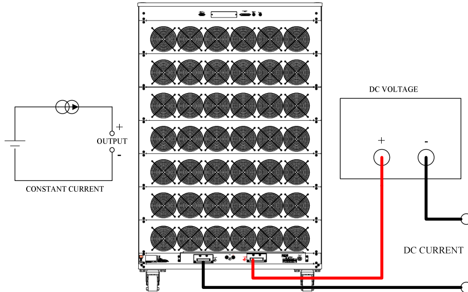
圖 5-8 固定電流源之連接圖
