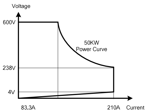
圖 1-1.1 36250高功率電子負載功率曲線圖
