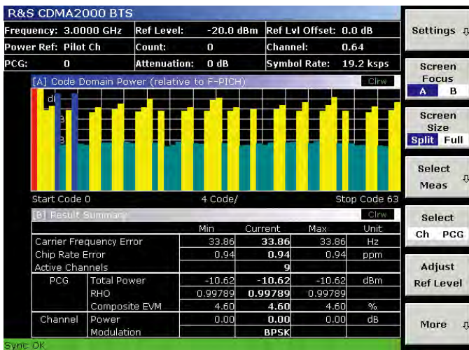
码域功率测量按照反向比特顺序显示激活和未激活的信道。结果汇总概述了信号主要测试参数，例如全部功率、信道功率、Rho和EVM。
