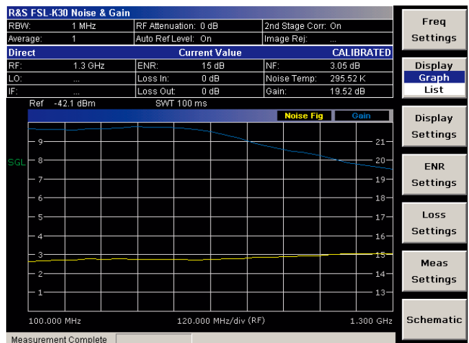
放大器测量
