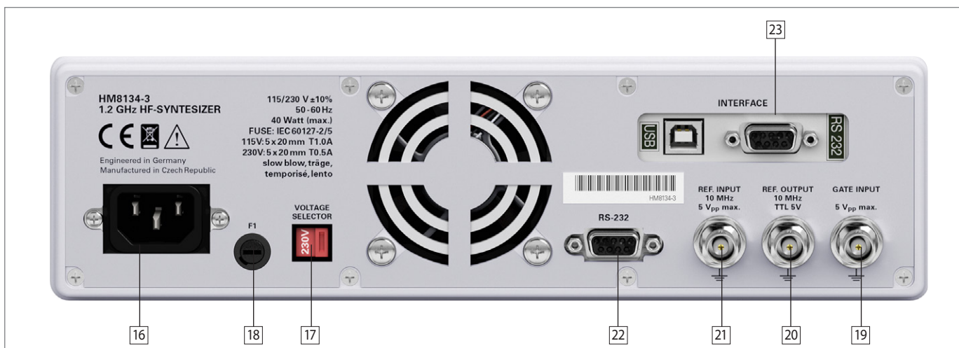
Abb. 2.2: Rückansicht des HM8134-3
