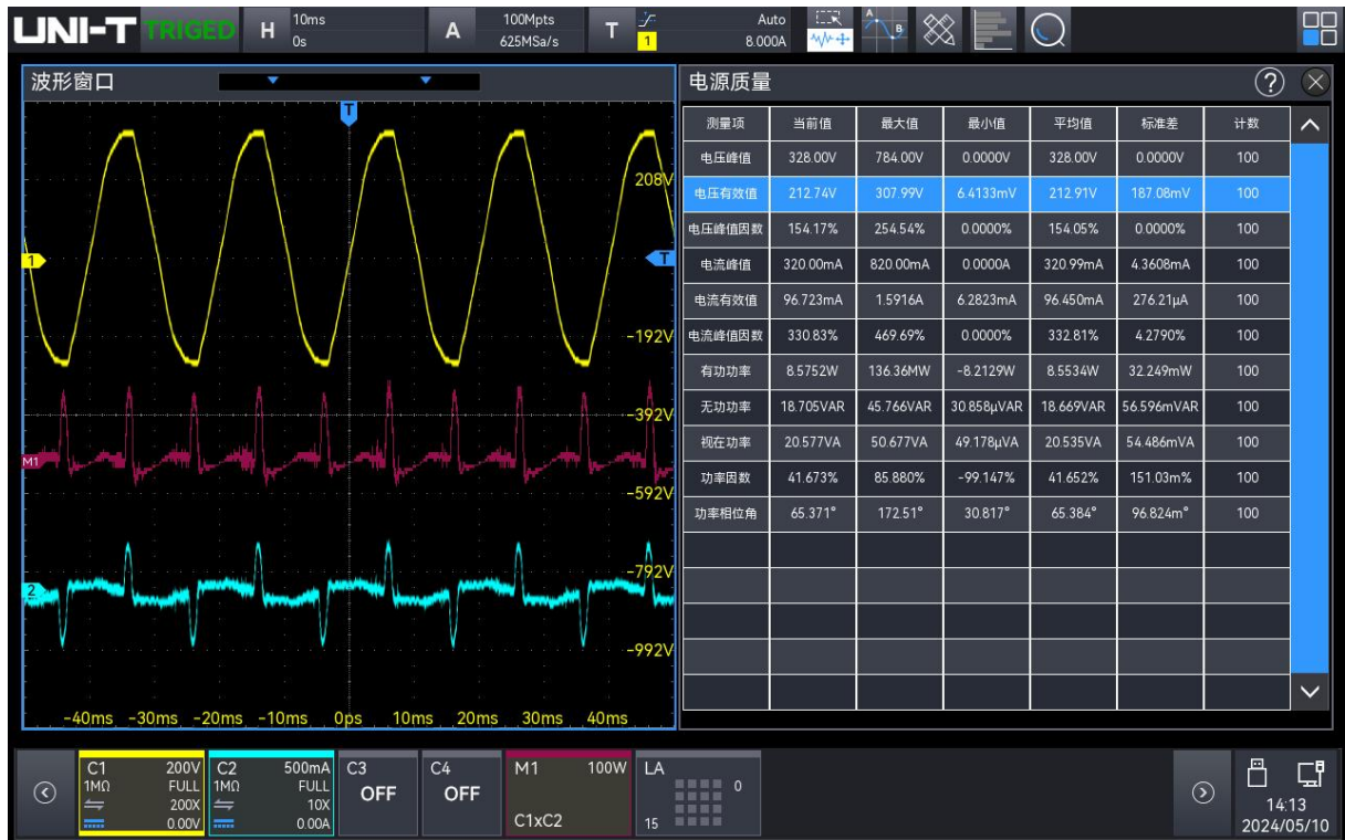
(12) 电源质量测试结果
