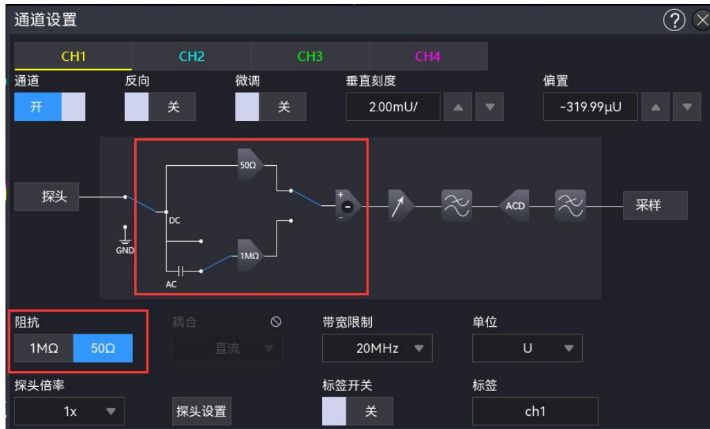
输入阻抗变更
