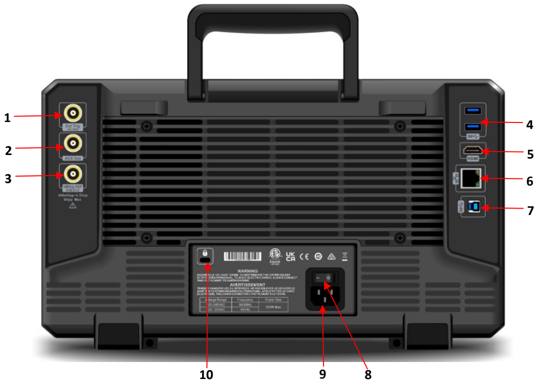
示波器后面板
