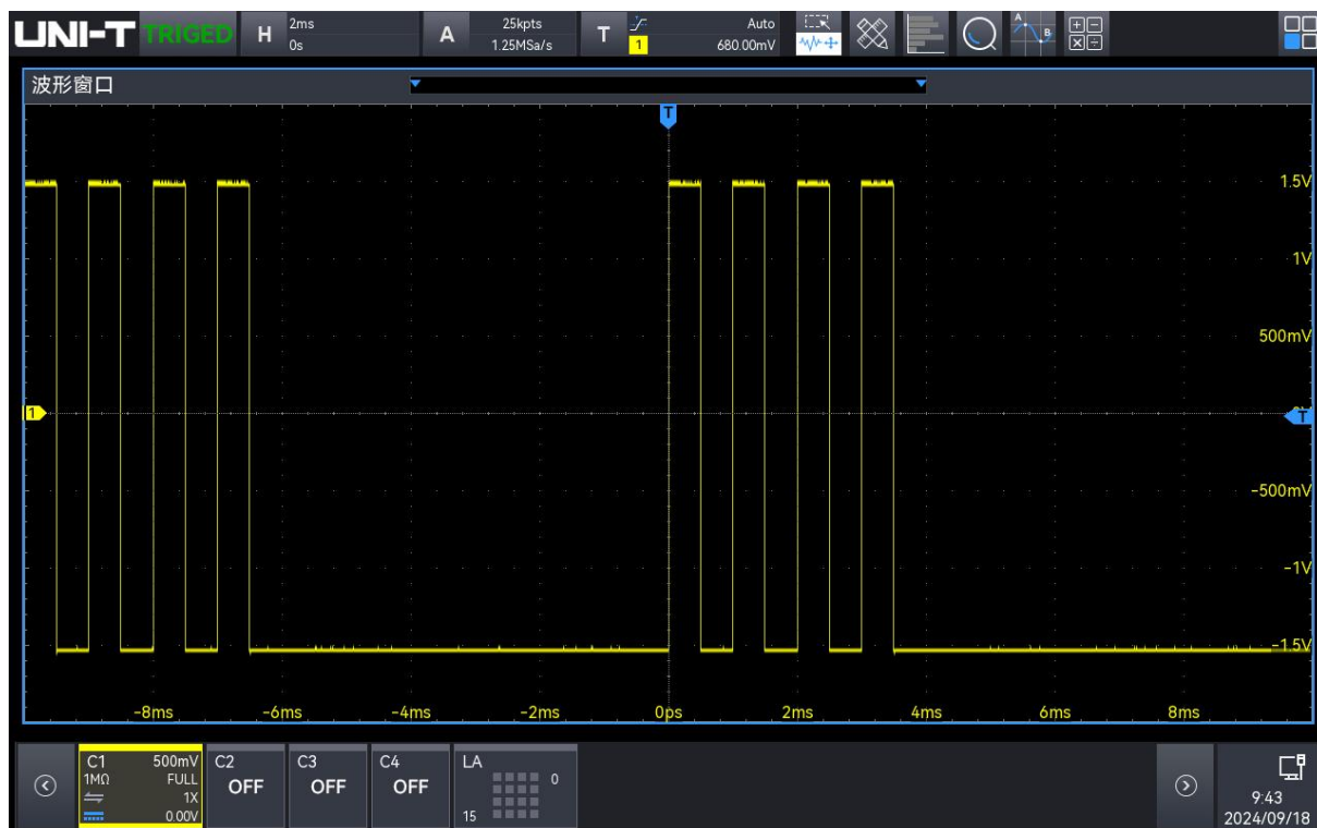
触发释抑示意图
