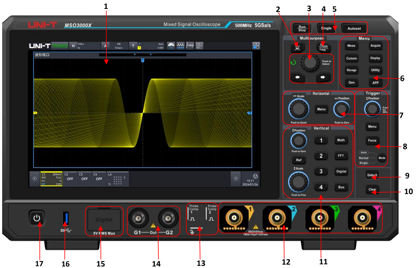
示波器前面板
