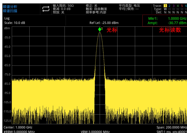
图 4-1: 标记光标读数
