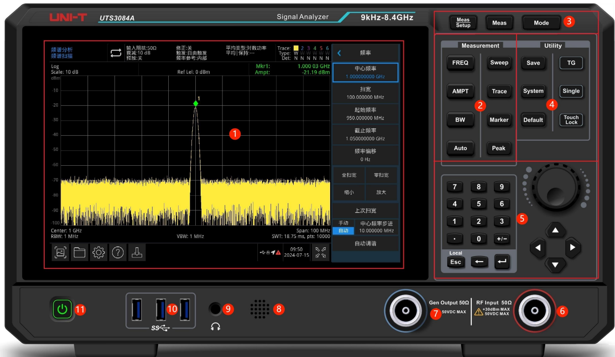
图 1-1: 前面板
