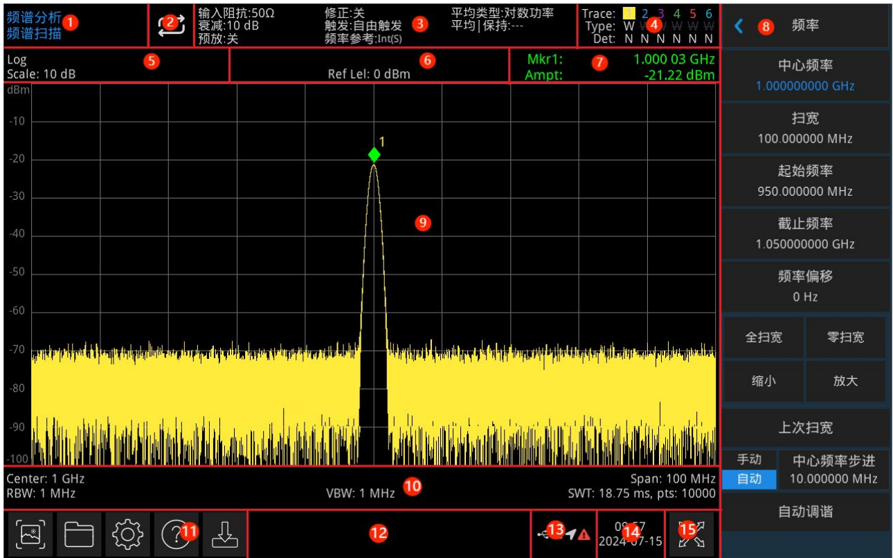
图 1-2: 用户界面
