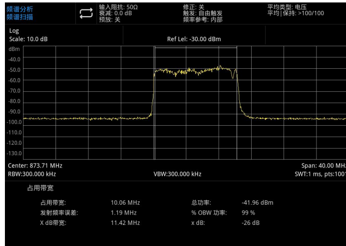
图 5-3: 占用带宽
