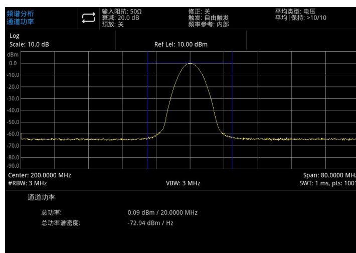
图 5-1: 通道功率
