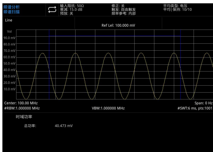
图 5-2：时域功率
