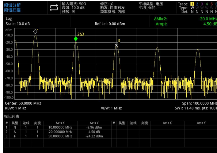
图 4-2：标记列表
