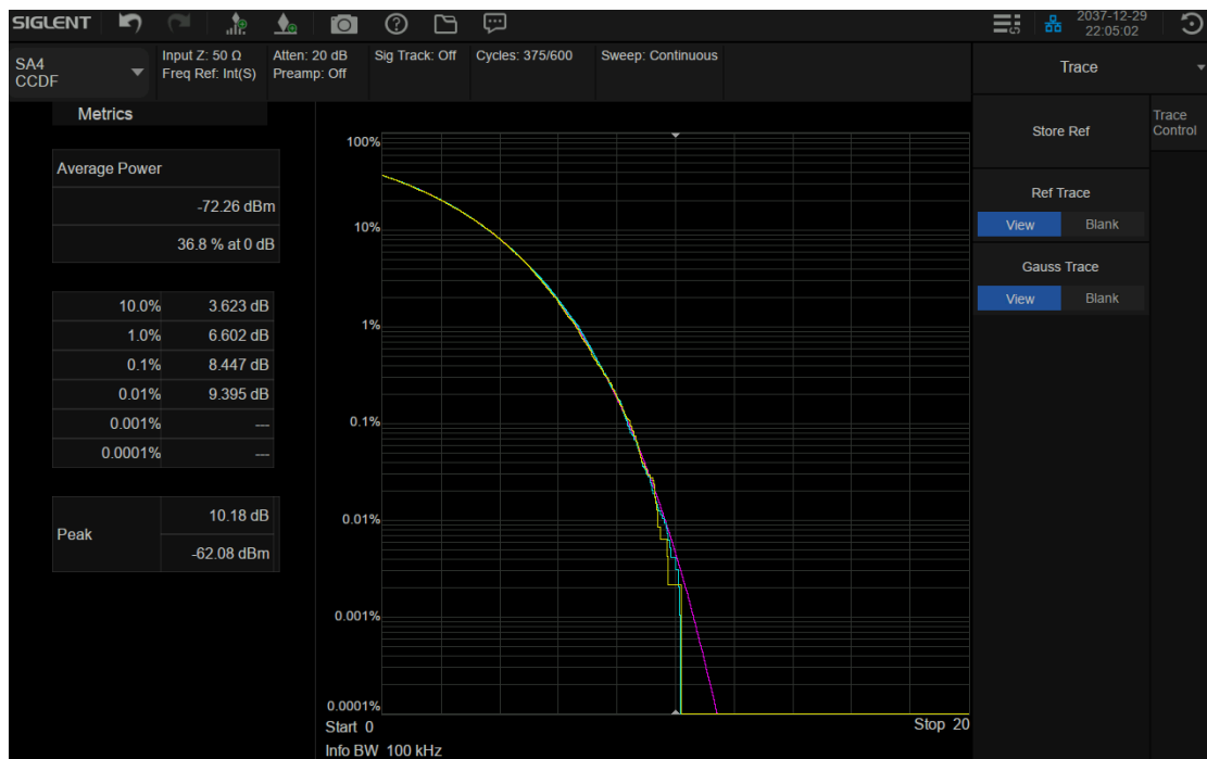
图 5-18 参考迹线示意图
