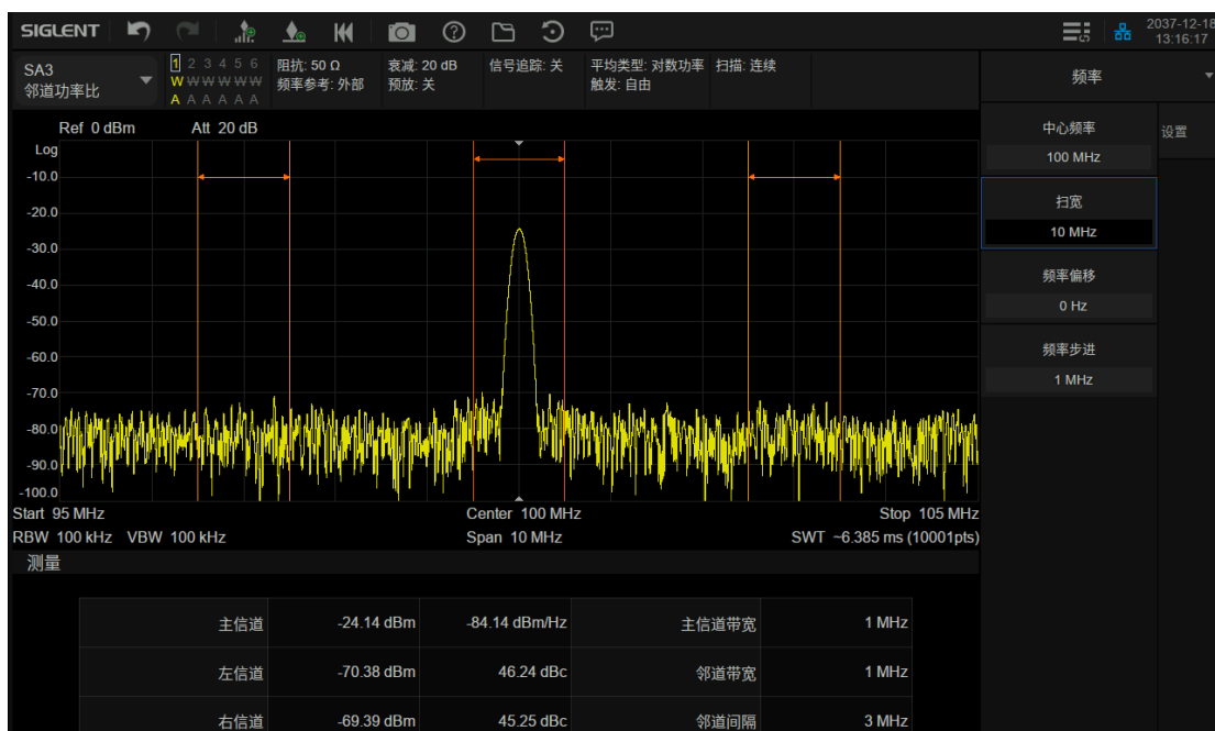
图 5-9 邻道功率比
