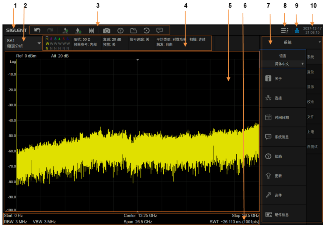
图 3-5 频谱分析仪模式用户界面
