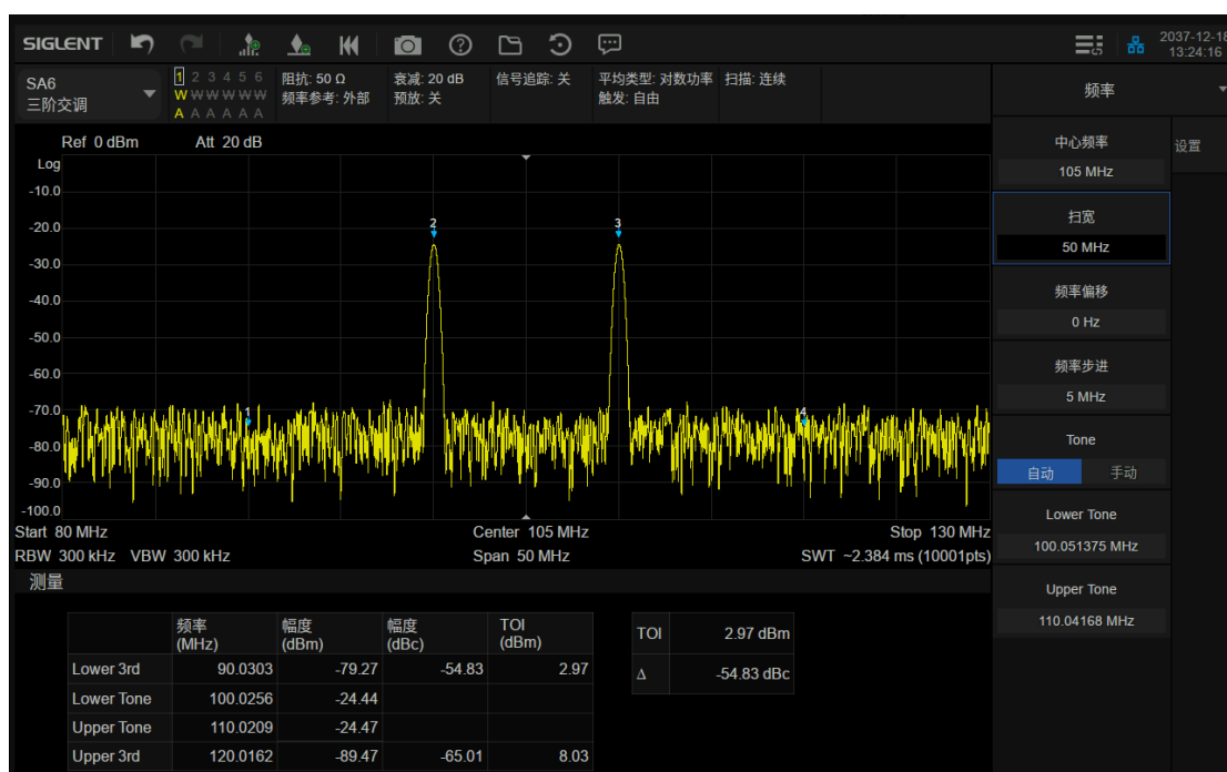
图 5-12 三阶交调
