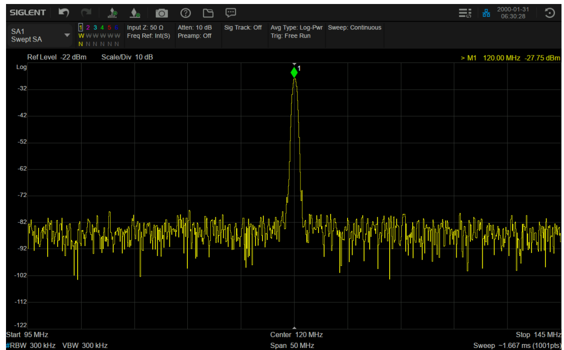
中频输出 1GHz RF 信号输入
