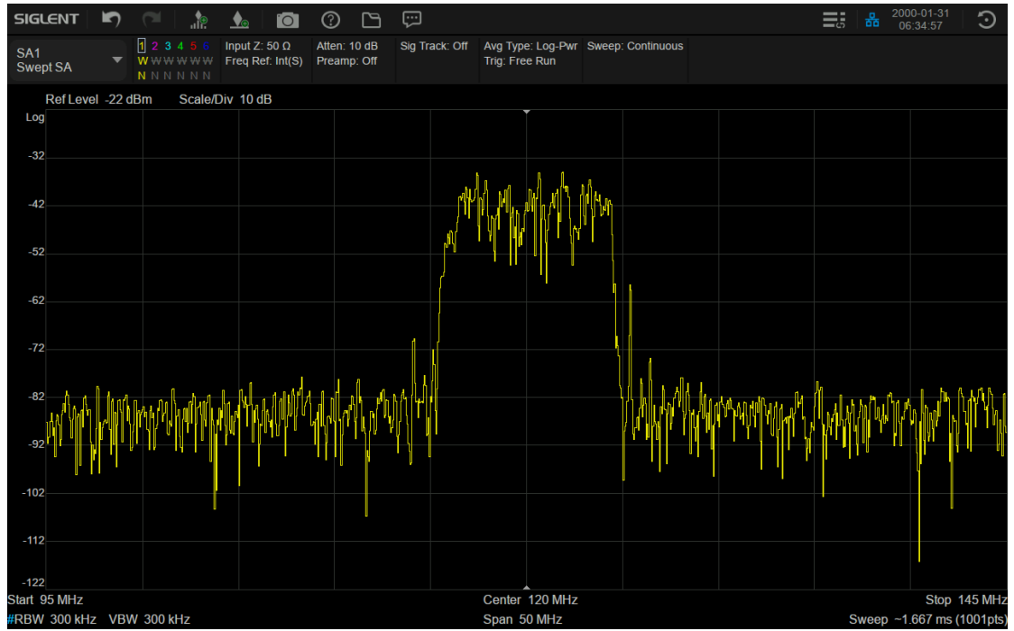
中频输出 3.5 GHz NR 信号输入
