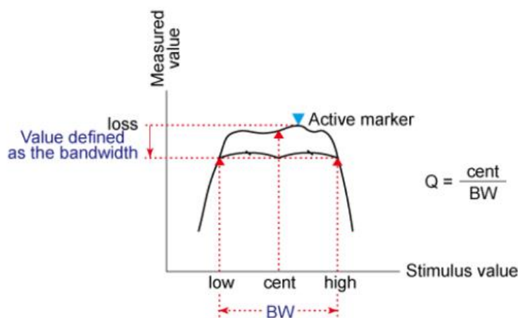
图 5-4 带宽的选择
