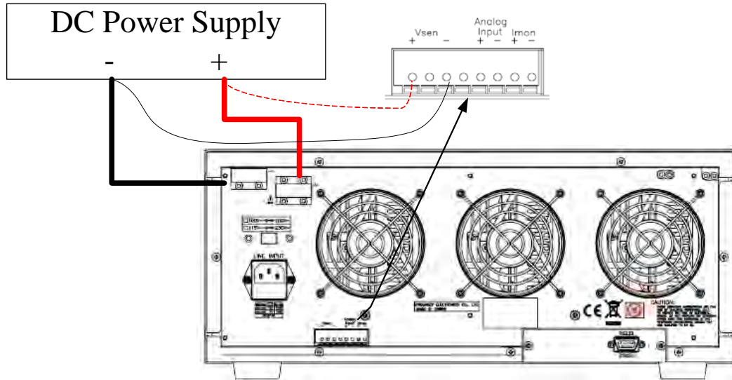
圖 3-3 典型 33501F 系列高功率電子負載連接方式
