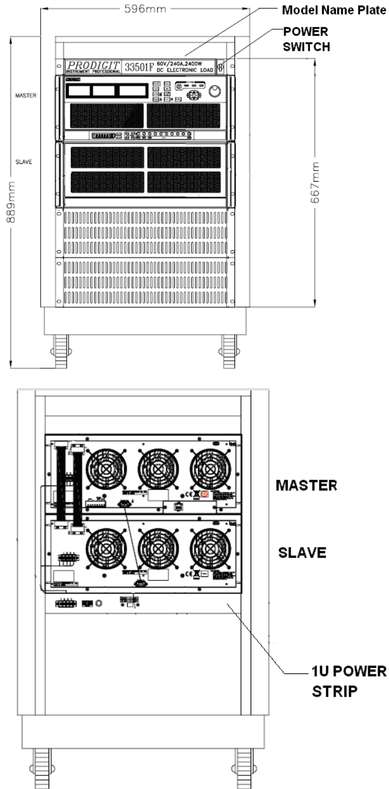
圖 3-2 33501F 系列高功率電子負載之前外後觀圖
