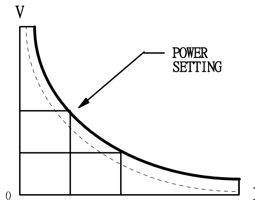
圖 1-5 固定功率模式特性圖
