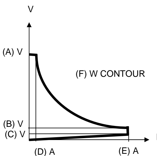
圖 1-1 33501F 高功率電子負載功率曲線圖
