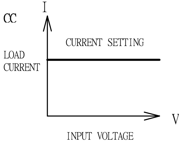
圖 1-2 固定電流模式特性圖
