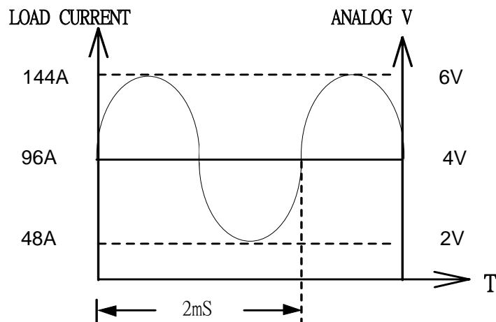
圖 3-7 負載電流之類比設定輸入
