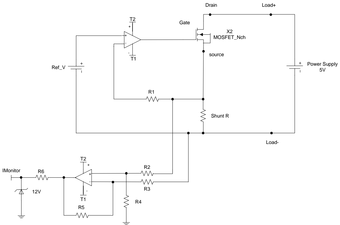
圖 3-4 33501F 系列 I-monitor 等效電路圖
