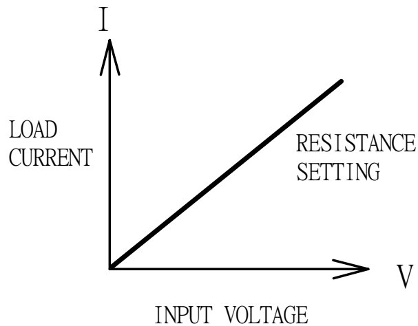
圖 1-3 固定電阻模式特性圖
