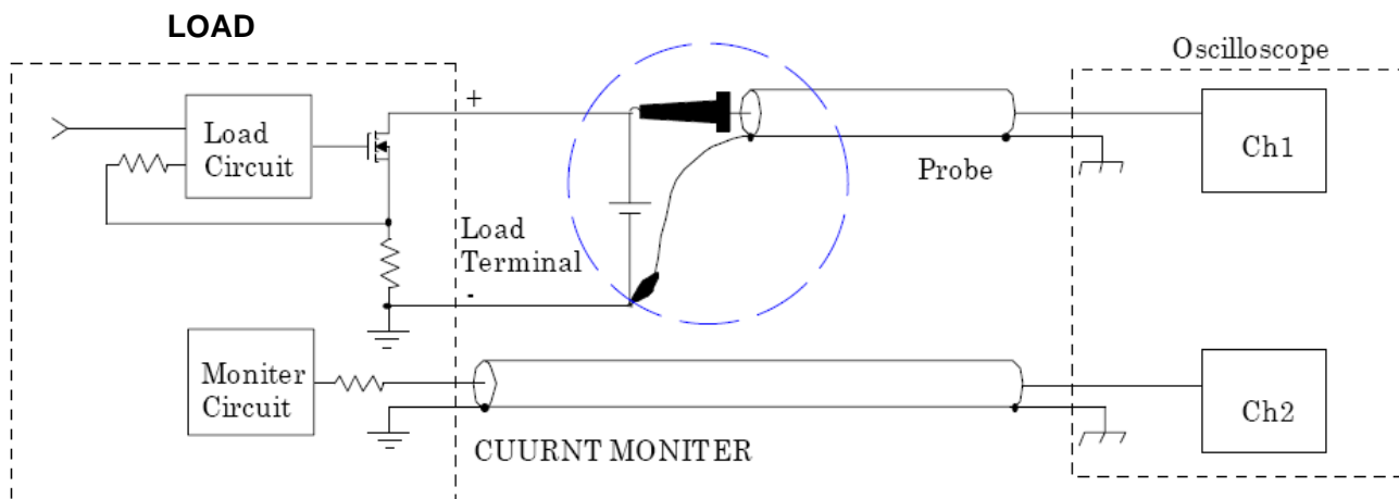
圖 3-5 示波器正確的連接圖
