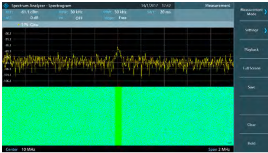
FPC-K55: 频谱瀑布图。
